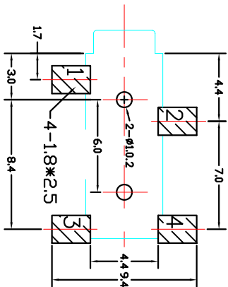
P.C.B. TERMINAL POSITION
