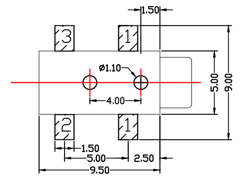
P.C.B TERMINAL POSITION
