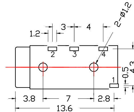
P.C.B TERMINAL POSITION
