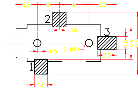
P.C.B. TERMINAL POSITION
